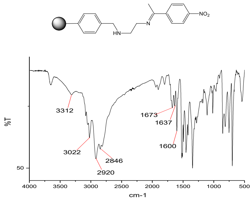
Figure S13. FT-IR spectrum of Med
