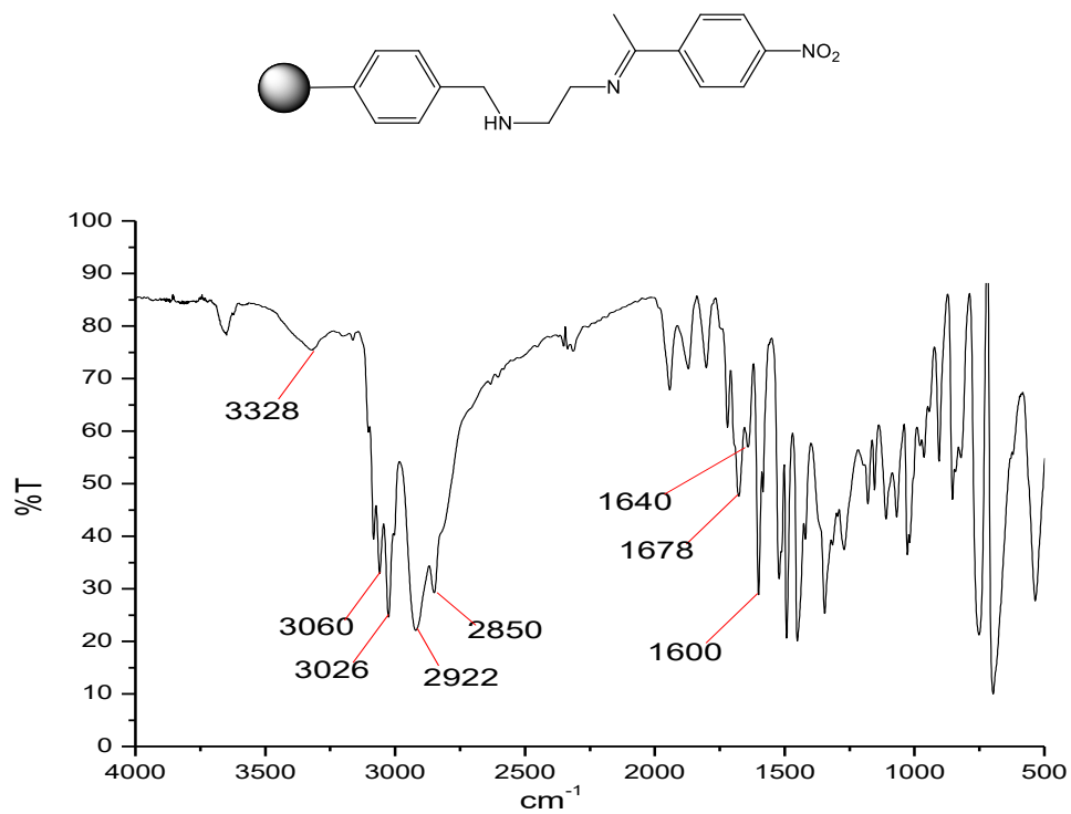
Figure S9. FT-IR spectrum of med
