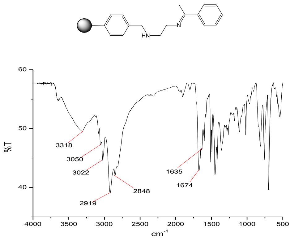
Figure S9. FT-IR spectrum of med
