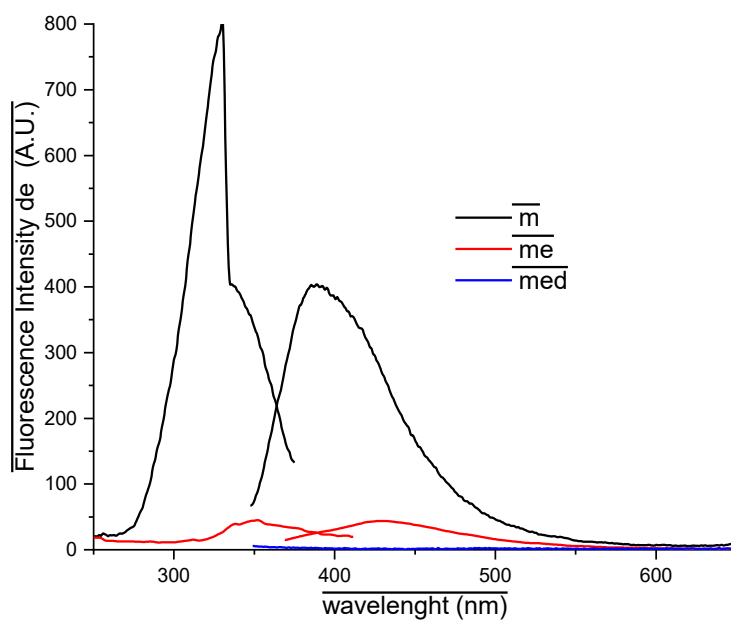
Figure S17. Fluorescence spectra of med
