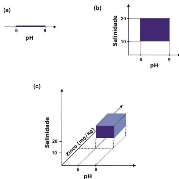
Figura 2. Representação esquemática do conceito de Nicho multidimensional. (a) Uma dimensão, pH; (b) Duas dimensões, pH e salinidade e em (c) Três dimensões, pH, salinidade e concentração de Zinco
