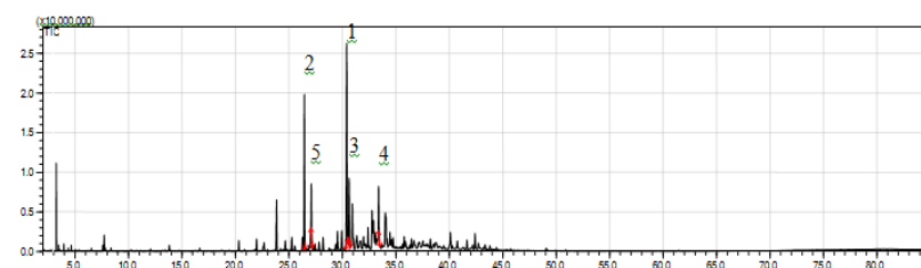
Figura 9S. Cromatograma do óleo essencial de folhas in natura de Cardiopetalum calophyllum coletadas em novembro/2014. 1 Espatuleno; 2 Germacreno-D; 3 Viridiflorol; 4 Acetato de (-) isolongifolol; 5 Germacreno-B
