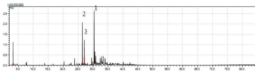
Figura 8S. Cromatograma do óleo essencial de folhas in natura de Cardiopetalum calophyllum coletadas em outubro/2014. 1 Espatuleno; 2 Germacreno-D; 3 Germacreno-B
