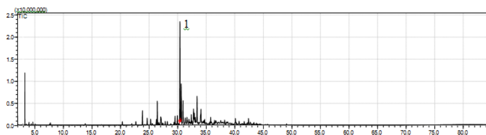
Figura 4S. Cromatograma do óleo essencial de folhas in natura de Cardiopetalum calophyllum coletadas em junho/2014. 1 EspatulenoI
