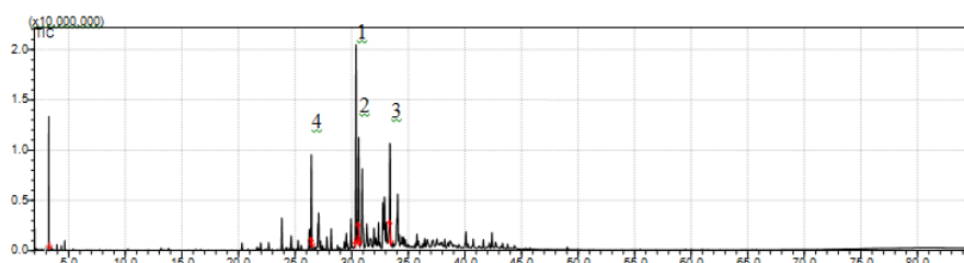
Figura 11S. Cromatograma do óleo essencial de folhas in natura de Cardiopetalum calophyllum coletadas em janeiro/2015. 1 Espatuleno; 2 Viridiflorol; 3 Acetato de (-) isolongifolol; 4 Germacreno-D.
