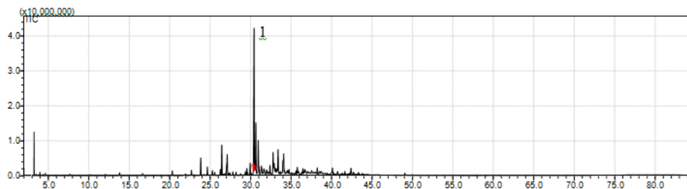
Figura 3S. Cromatograma do óleo essencial de folhas in natura de Cardiopetalum calophyllum coletadas em maio/2014. 1 EspatulenoI
