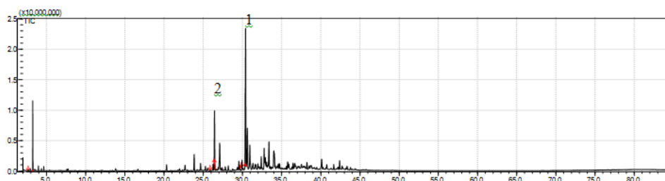
Figura 6S. Cromatograma do óleo essencial de folhas in natura de Cardiopetalum calophyllum coletadas em agosto/2014. 1 EspatulenoI; 2 Germacreno-D
