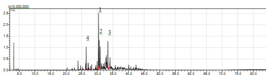
Figura 10S. Cromatograma do óleo essencial de folhas in natura de Cardiopetalum calophyllum coletadas em dezembro/2014. 1 Espatuleno; 2 Viridiflorol; 3 ent-espatuleno; 4 Germacreno-D
