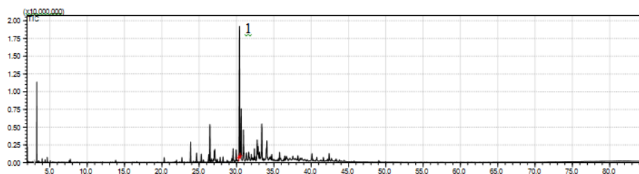
Figura 5S. Cromatograma do óleo essencial de folhas in natura de Cardiopetalum calophyllum coletadas em julho/2014. 1 EspatulenoI
