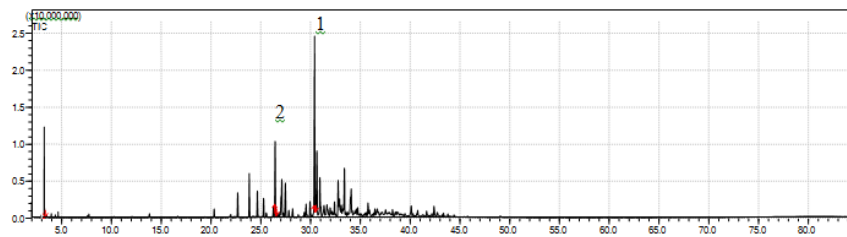
Figura 7S. Cromatograma do óleo essencial de folhas in natura de Cardiopetalum calophyllum coletadas em setembro/2014. 1 Espatuleno; 2 Germacreno-D
