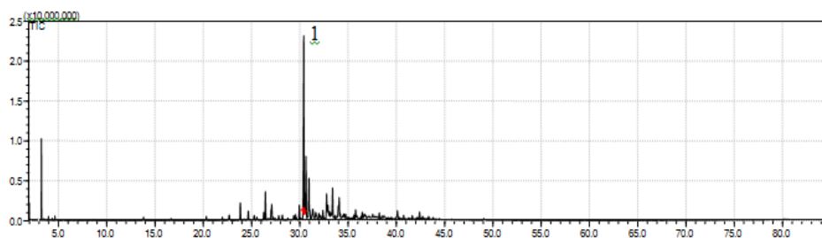
Figura 2S. Cromatograma do óleo essencial de folhas in natura de Cardiopetalum calophyllum coletadas em abril/2014. 1 Espatuleno
