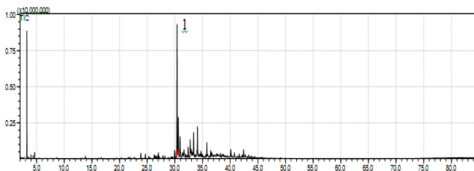
Figura 1S. Cromatograma do óleo essencial de folhas in natura de Cardiopetalum calophyllum coletadas em março/2014. 1 Espatuleno
